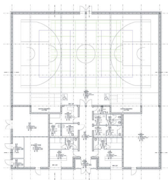
Der Grundriss zeigt die Einteilung der Einfeldsporthalle mit dem Sozialtrakt.
